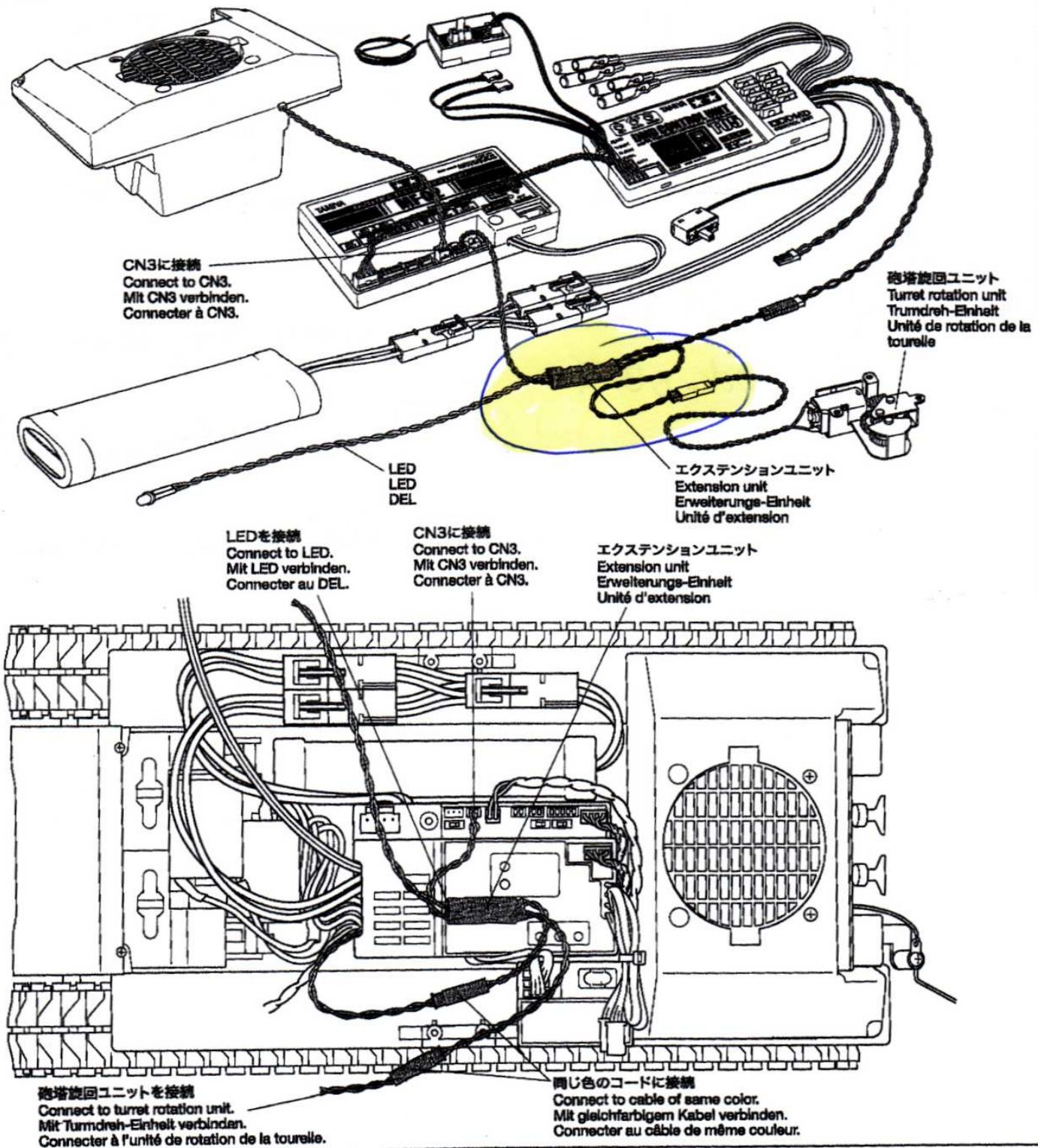
ユニット配線図 Circuit diagram Schaltbild Schéma du circuit
